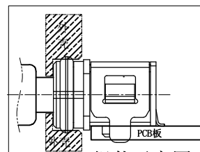
组装示意图
