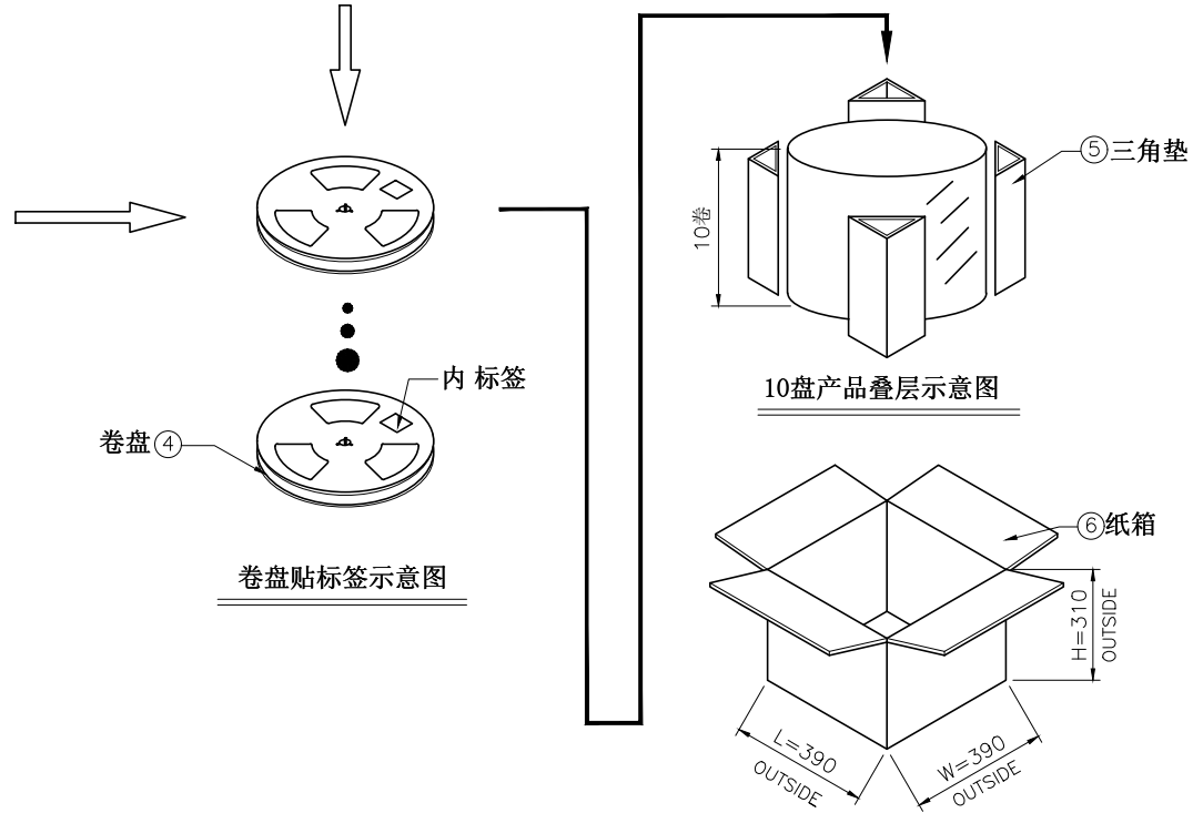
包装示意图
