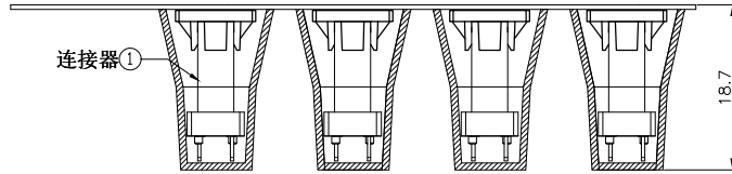
产品入载带示意图
