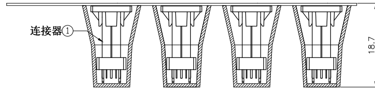
产品入载带示意图
