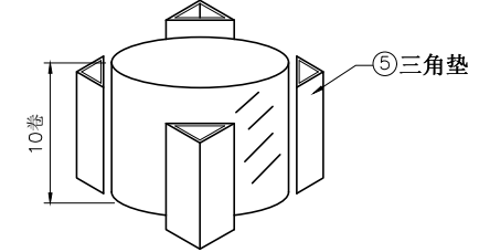
10盘产品叠层示意图
