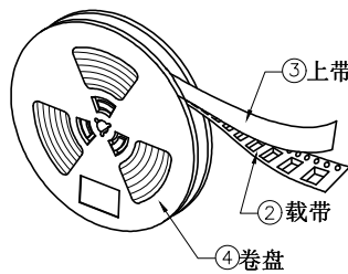
卷盘示意图
