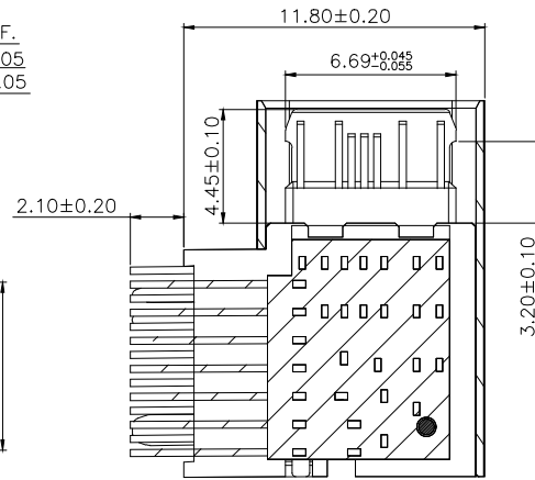
剖视图
