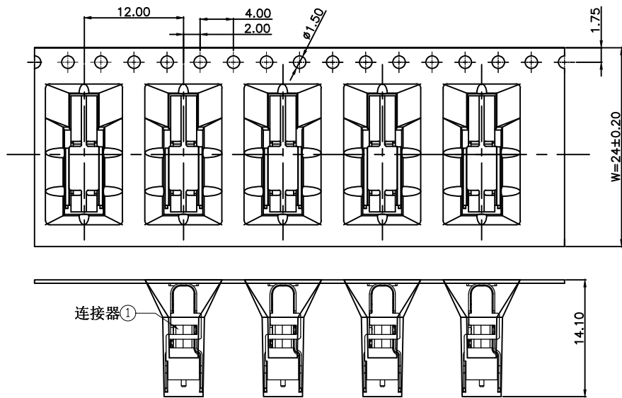
产品入载带示意图
